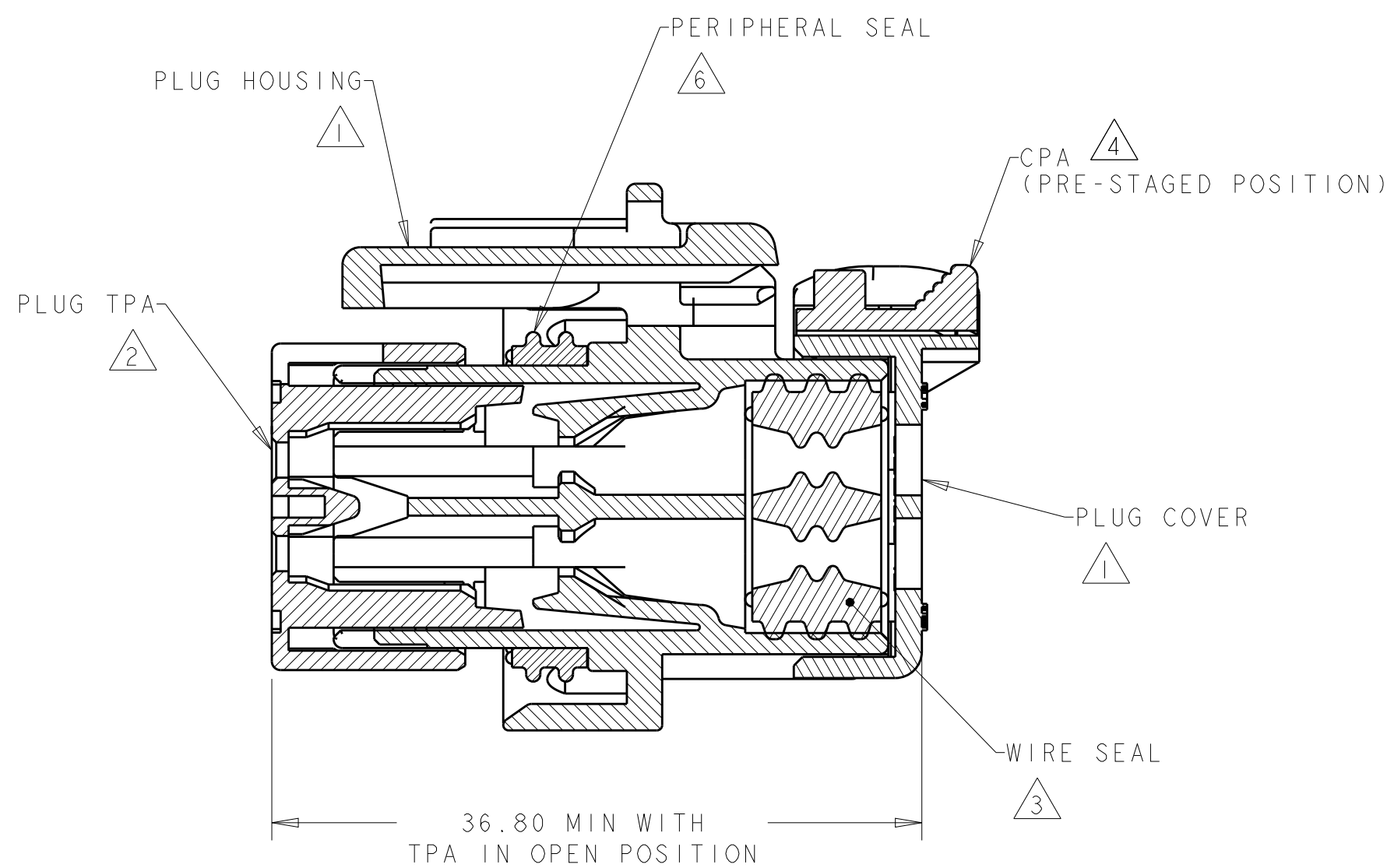
SECTION A-A
