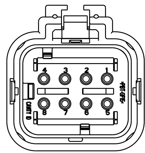
776494-4 SCALE 2:1
